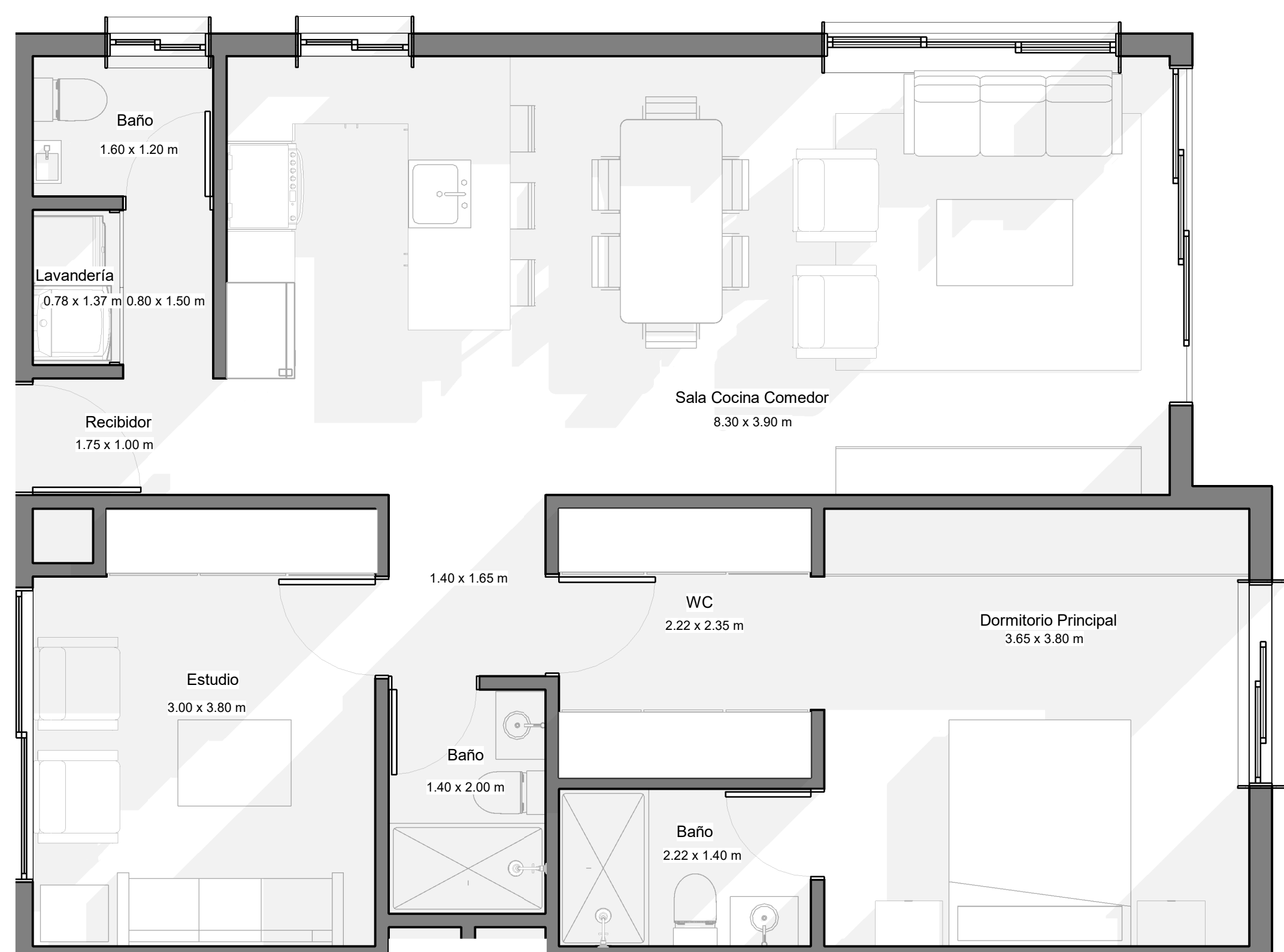
APARTAMENTO Tipo 101 1:40
