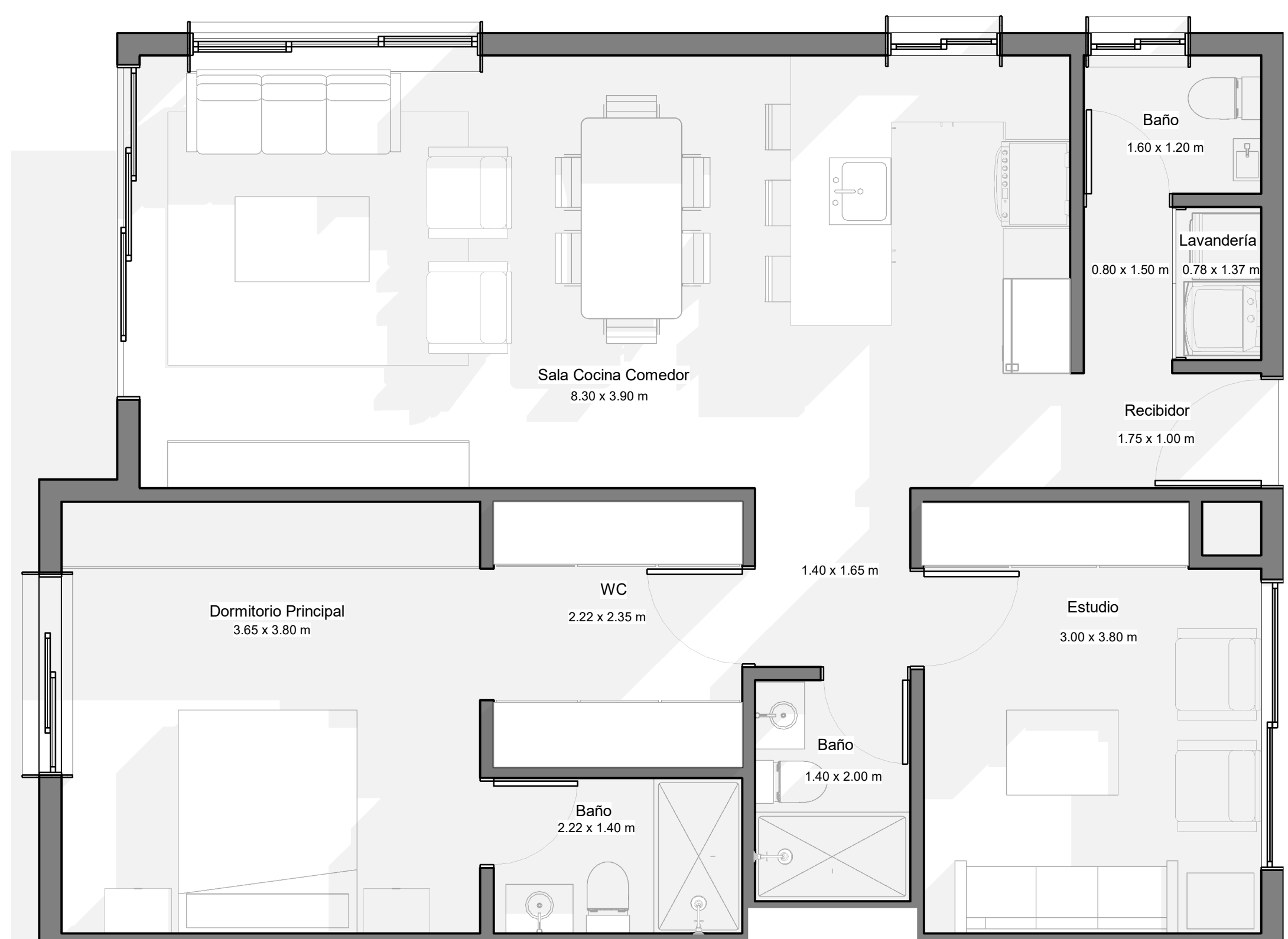
APARTAMENTO Tipo 104 1:40
